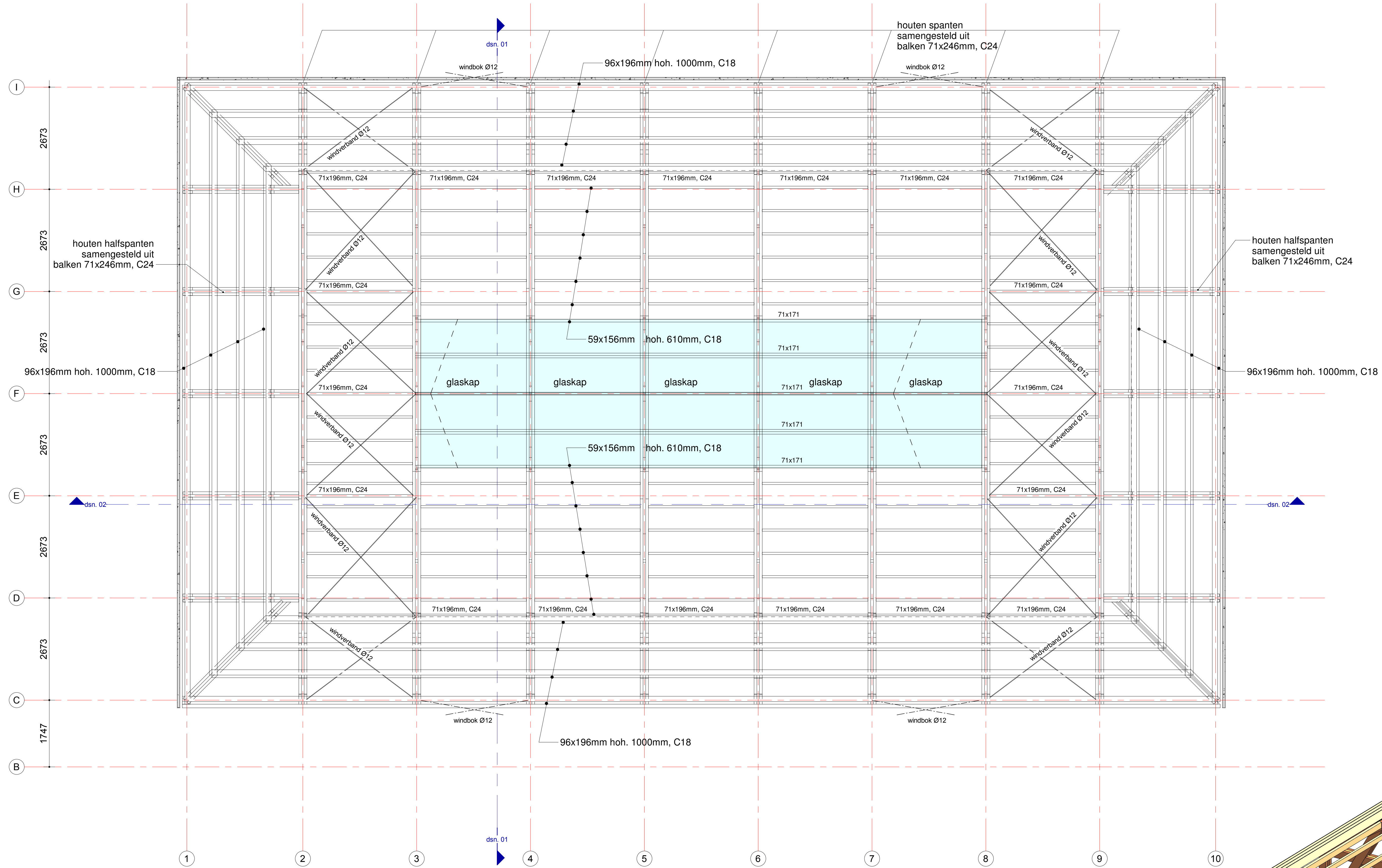
Dakconstructie 1:50
